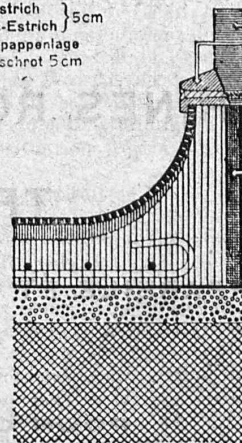
Patenterte „Isolaphon“-Unterlagsboden
