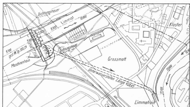
Fig. 1. — Plan de situation de l'aménagement hydraulique de Wettingen. Echelle 1 : 8000.
