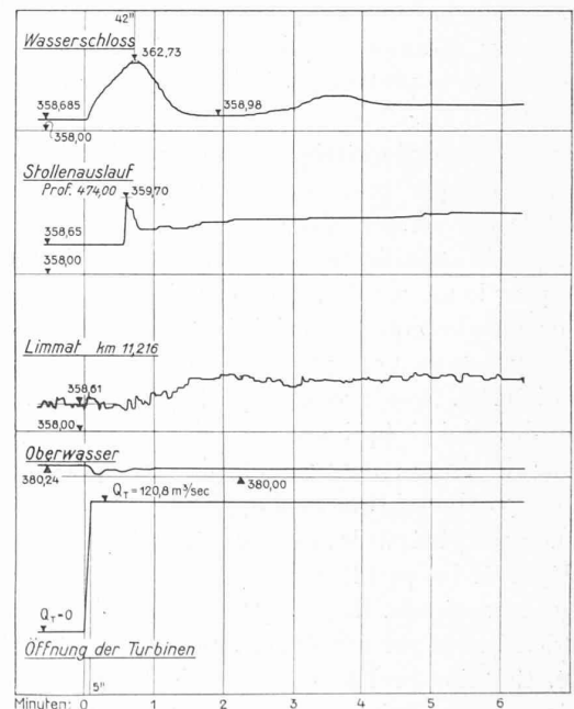
Fig. 5. — Diagramme multiple, enregistré au chronographe d'Amsler sur le modèle, lors d'une ouverture des 3 turbines (Q T = 0 à 120 m 3 : s) en 5 sec., par une crue exceptionnelle de la Limmat (Q L = 500 m 3 : s).
