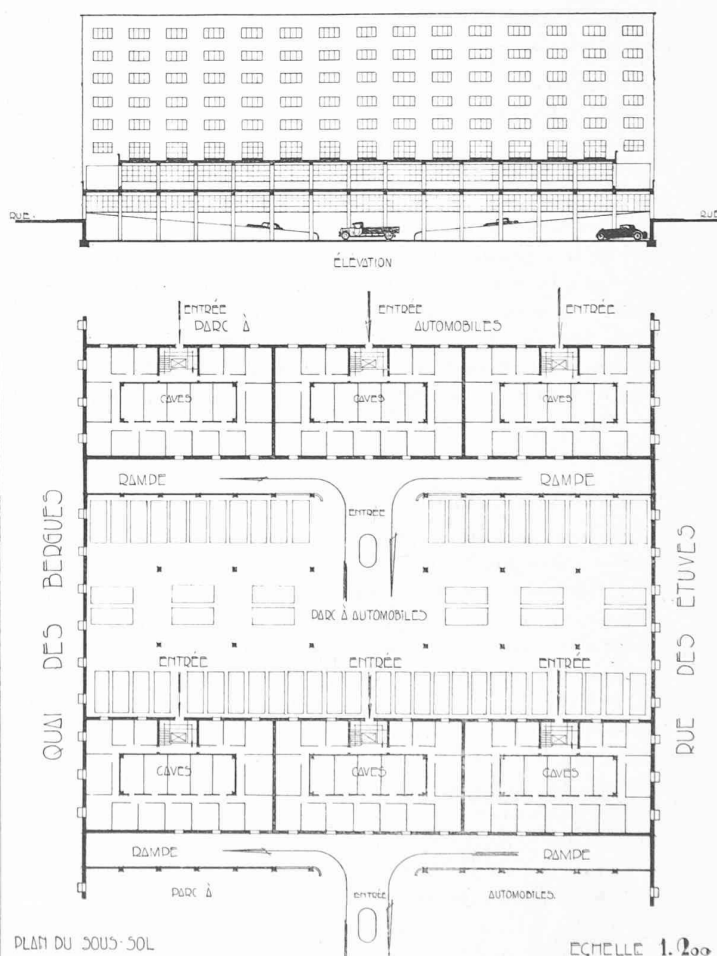
Fig. 4. — Plan et coupe indiquant les particularités des parrés à autos, en sous-sol.
