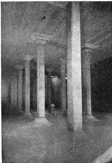
Grand réservoir du Gutsch, Lucerne (8000 m 3 ).
