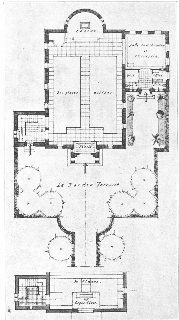
Plan du temple et de la galerie — 1 : 300.
