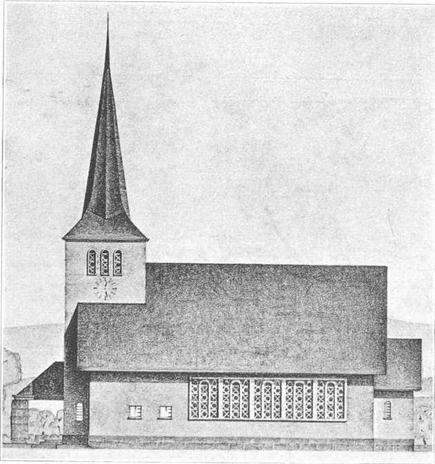
Façade est — 1 : 300.
