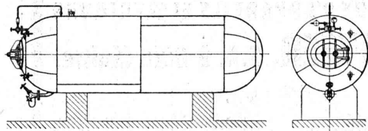
Tank à moûts, en acier inoxydable. Pression d'acide carbonique : 7 atm.
