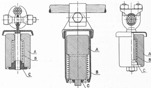
Fig. 5. — Trois exemples d'exécution d'amortisseurs à ressort.
