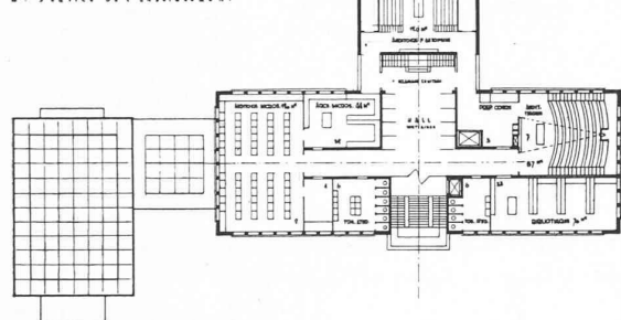
PLAN DU PREMIER ETAGE A : SERVICES DE L'ENSEIGNEMENT
