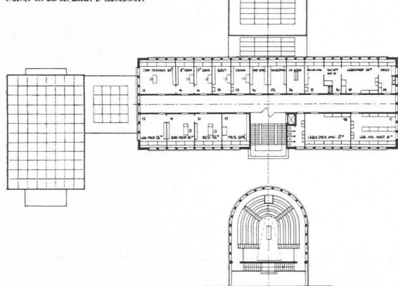
PLAN DU DEUXIEME ETAGE SERVICES DES BIOPHYSIQUES, QUARTIER ET LABORATOIRES
