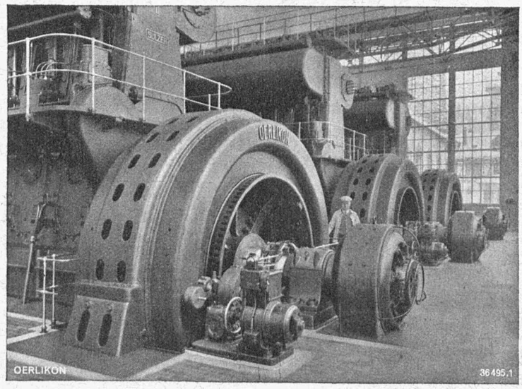
OERLIKON 36 495.1 Centrale Diesel-électrique de Kubel (St-Gall), 3 alternateurs triphasés de 6250 kVA chacun.
