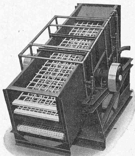
Cribles à oscillations libres. Nouvel appareil de tamisage pour sable et gravier, ainsi que pour toutes applications industrielles.
