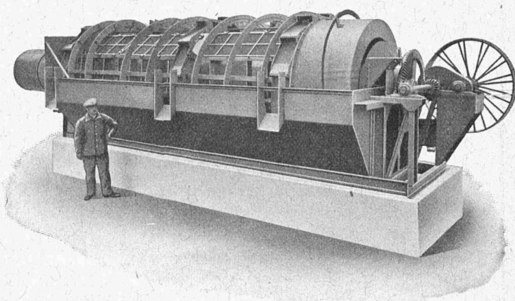
Laveuse-trieuse à bac pour sable et gravier. La machine idéale pour un triage impeccable et un lavage irréprochable.
