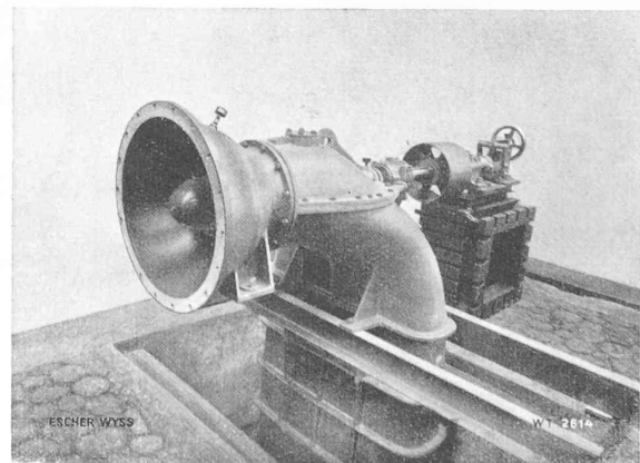
Fig. 6. — Turbine Kaplan à distributeur axial fixe, placée au bout d'une conduite. H = 6,5 m P = 66 ch n = 890 t : mn
