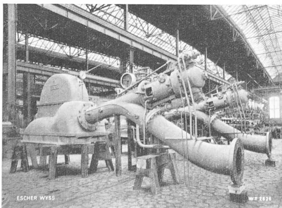
Fig. 4. — Turbines Pelton de la centrale de Pallivasal. H = 604 m P = 6570 ch n = 750 t : mn
