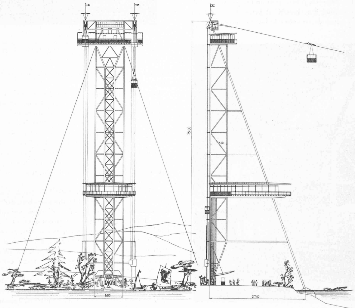
Fig. 4. — Pylône du téléphérique.
