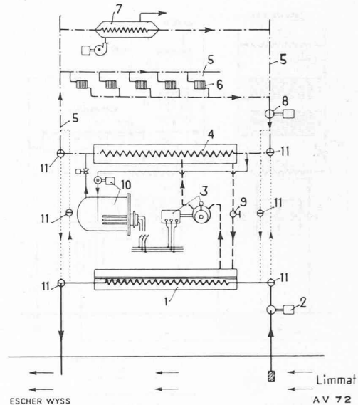
Fig. 14. — Schéma de l'installation de chauffage de l'Hôtel de Ville de Zurich, par pompe à chaleur.
