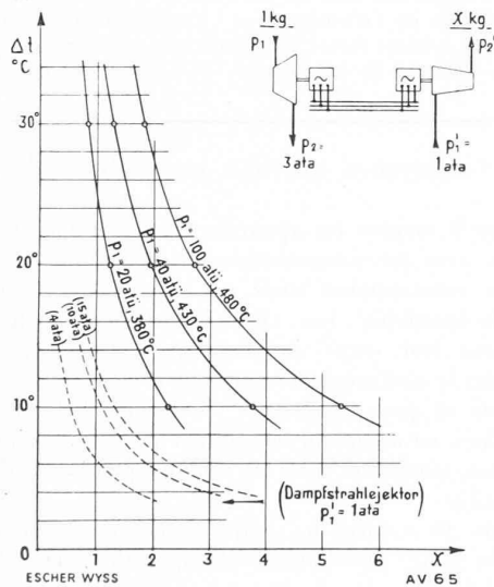
Fig. 11. — Comparaison de groupes turbo-compresseur pour formation de vapeur. ata = at. abs. atu = at. eff. Dampfstrahlejektor = éjecteur de vapeur.
