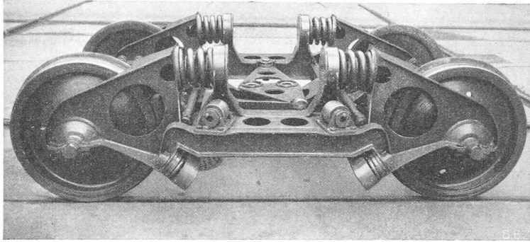
Fig. 8. Bogie porteur du train léger du chemin de fer BSB, à roues indépendantes.
