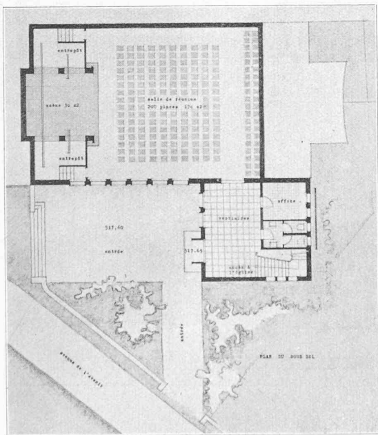
Plan du sous-sol. — Echelle 1 : 400.
