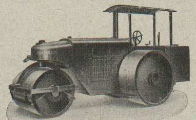
Rouleau-compresseur trijante
