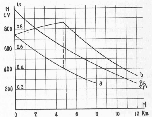
Fig. 1. — Variation de la densité de l'air \frac{\rho}{\rho_0} et puissance d'un moteur en fonction de l'altitude H : a) sans compresseur — b) avec compresseur.
