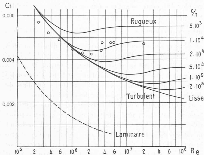
Fig. 6. — Coefficient de frottement C_f pour une plaque mince lisse ou rugueuse, en fonction du nombre de Reynolds Re , h désigne la hauteur moyenne des rugosités et c la largeur de la plaque ou la corde de l'aile.
