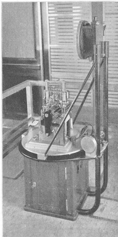
Fig. 36. — Appareil Hallade.
