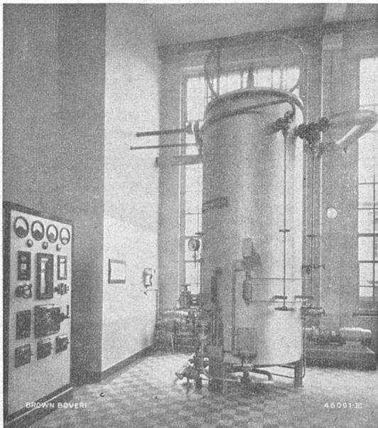
Chaudière électrique de 2000 kw, 10 000 V, 17 kg/cm 2 ats.
