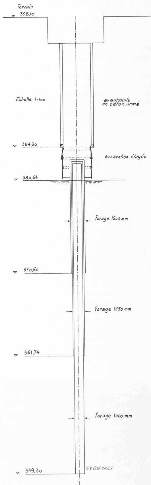
Fig. 5. — Schéma de l'ouvrage en cours d'exécution.
