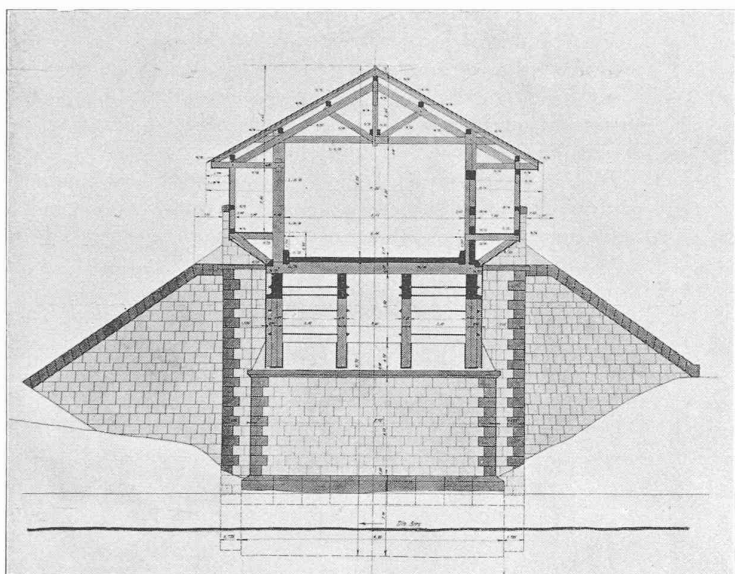
Fig. 2. — Coupe transversale.
