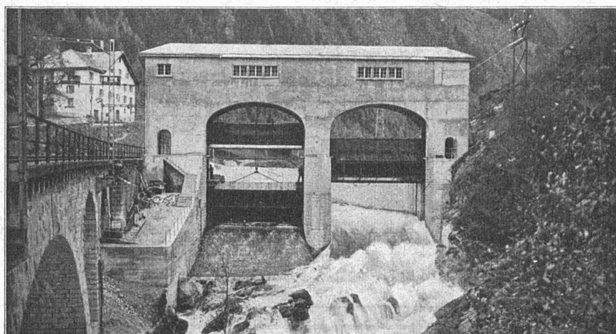
Barrage automatique de Piottino à Rodi-Fiesso.
