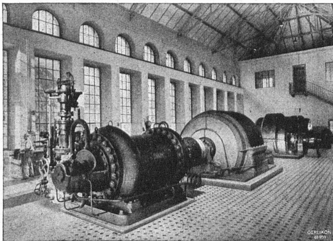
Station de pompage pour accumulation de la S. A. Illsee-Turtmann, Lausanne.
