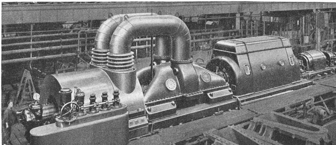
Groupe turbo-générateur à deux cylindres et condenseur axial 22000/27000 kW, 3000 t/min, 31250 kVA, 11000 V, génératrice pour services auxiliaires adossée.
