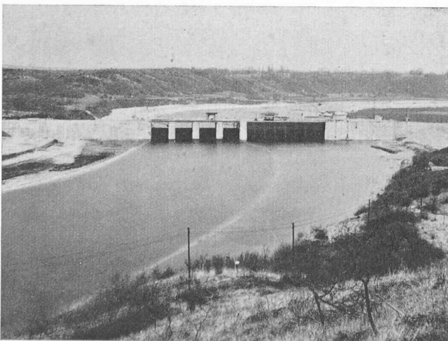
Fig. 39. — Vue générale de l'amont au début de la mise en eau. (A comparer à fig. 23 et 1.)
