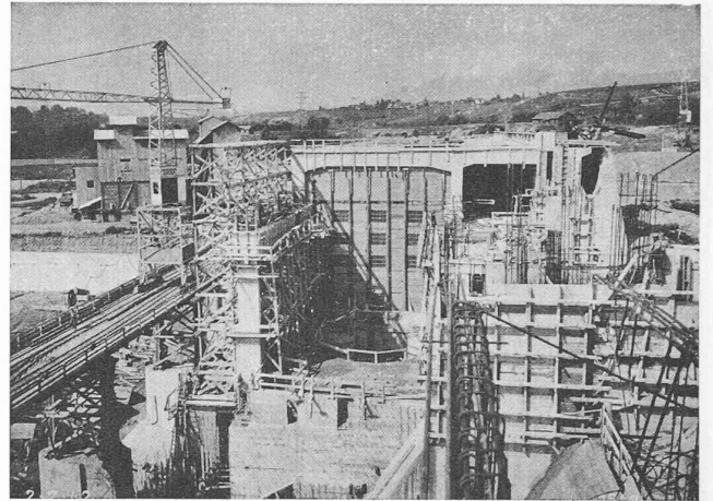
Fig. 38. — Chantier de la salle des machines et ouvrages d'entrée, vu du barrage.
