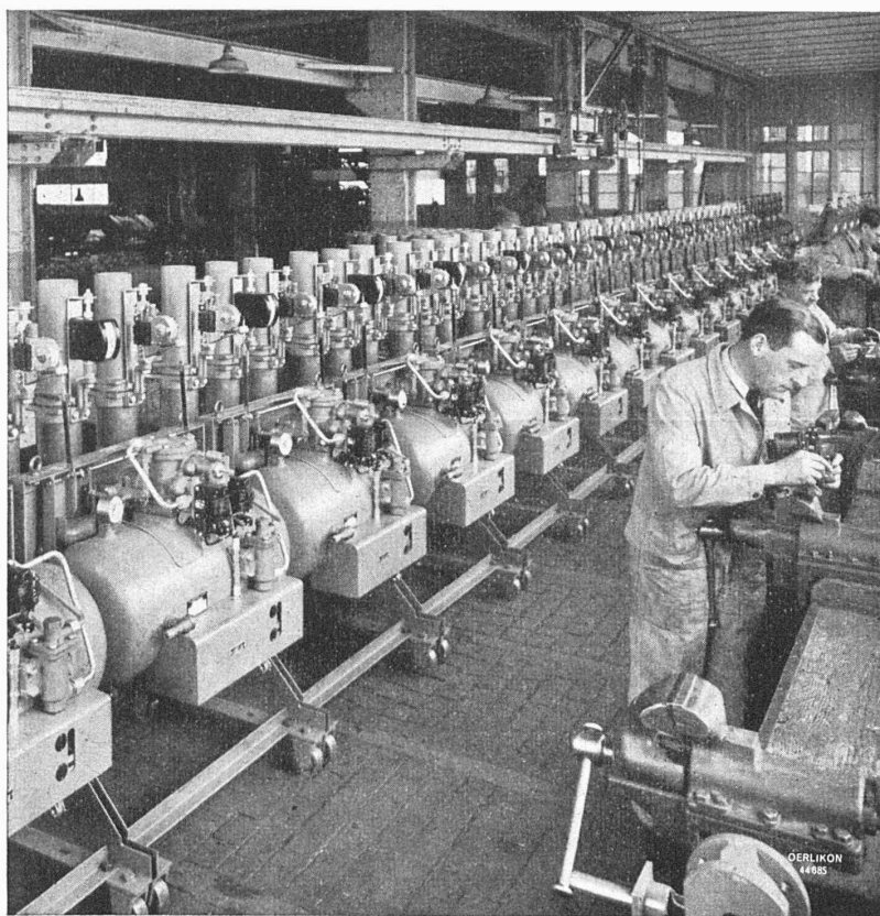
Montage de disjoncteurs rapides à air comprimé Oerlikon.
