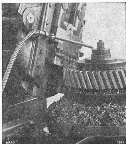
Taillage d'un engrenage à denture héliçoïdale sur machine MAAG
