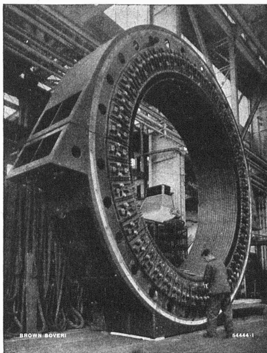
Travaux d'usinage du stator d'un alternateur de grande puissance.
