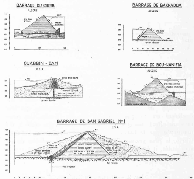
Fig. 4. — Profils des barrages algériens du type digue en enrochements.
