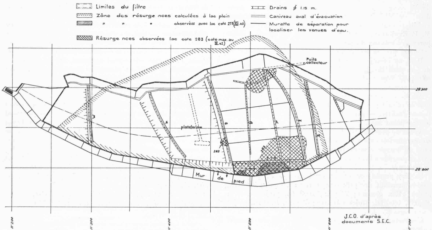
Plan de situation. Fig. 15. — Observation des zones de résurgence des pertes.
