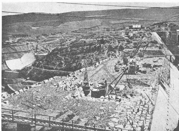
Fig. 5. — Barrage en enrochements du Ghrib.
