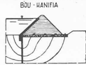
FILTRE HORIZONTAL CONTINU
