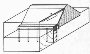
Fig. 14. — Différents types de filtres.
