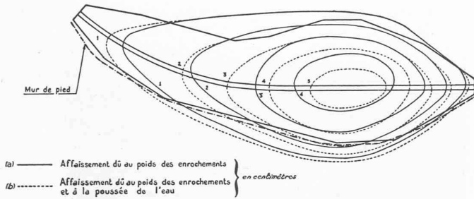
Fig. 9. — Les prévisions de tassement du terrain. Max. 4 cm à lac vide. Max. 5 cm à lac plein. D'après Rapport Congrès des grands barrages. Washington. 1936
