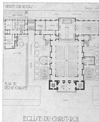
Plan — Echelle 1 : 1500.
