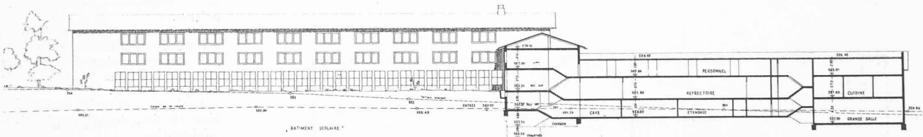
Vue du sud-est et coupe — Echelle 1 : 800.
