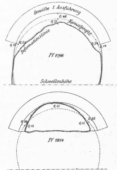
Fig. 4. — Tunnel du Saint-Gothard. Déformation du revêtement au km 2,796 et 2,814 deux mois après son exécution.
