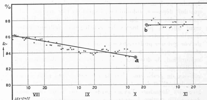
Fig. 14. — Variation du rendement journalier moyen de l'usine d'Innertkirchen, calculé d'après les lectures des compteurs de kWh et des débitmètres relevés en service (d'août à novembre 1944).
