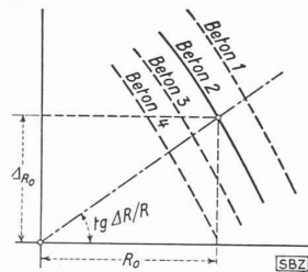
Fig. 39. — Courbes expansives dynamiques des divers bétons.
