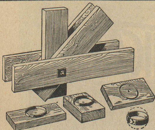
Ringdübel + Patent Assemblage de charpente en bois
