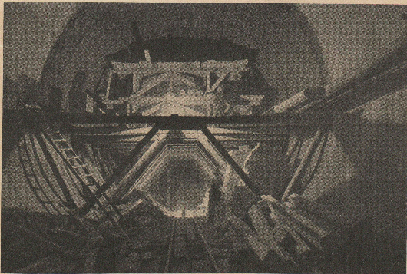
Usine électrique de Lavey. — Revêtement étanche de la galerie d'aménée sous pression, exécuté en asphalte souple « système Hirschy ».
