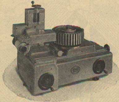
f Appareil MAAG, type FP-30 à contrôler le profil de dents d'engrenages droits ou hélicoïdaux.
