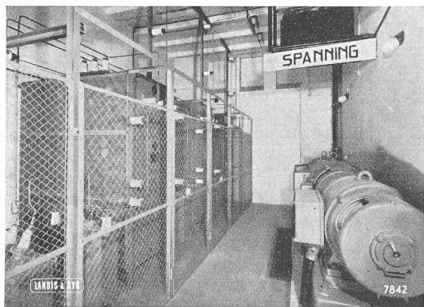
Fig. 16. — Groupe convertisseur de l'installation de télécommande des GEB Dordrecht (Hollande) avec ses 400 doubles-commandes. (Portées plus tard à 600.)
