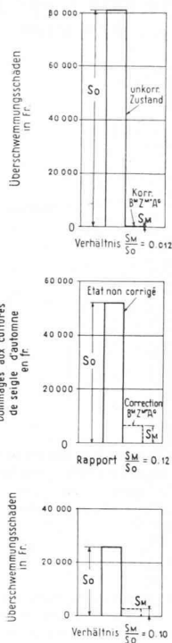
Fig. 7. — Effets de la correction sur les dommages dus aux inondations. Hautes eaux de 1944.
