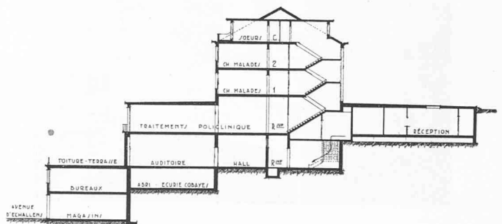
Fig. 2. — Coupe du nouvel hôpital.
