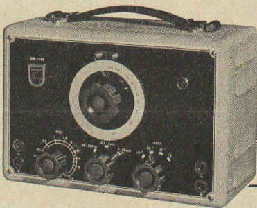
Générateur RC, GM 2315
