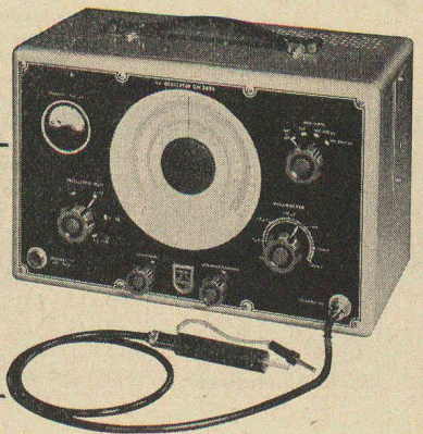
Oscillateur HF, GM 2883/93
