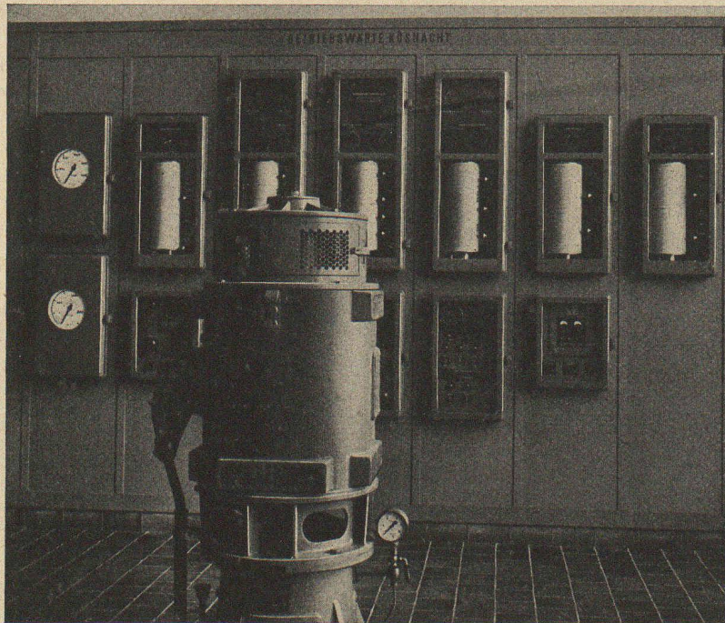
Service des Eaux de Küsnacht (ZH). Station de pompage au lac. Poste central de télémesure et de télécommande.
