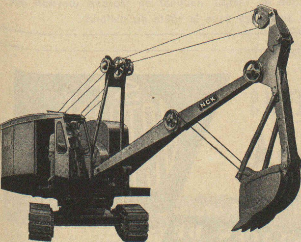
Equipement rétro-caveur
