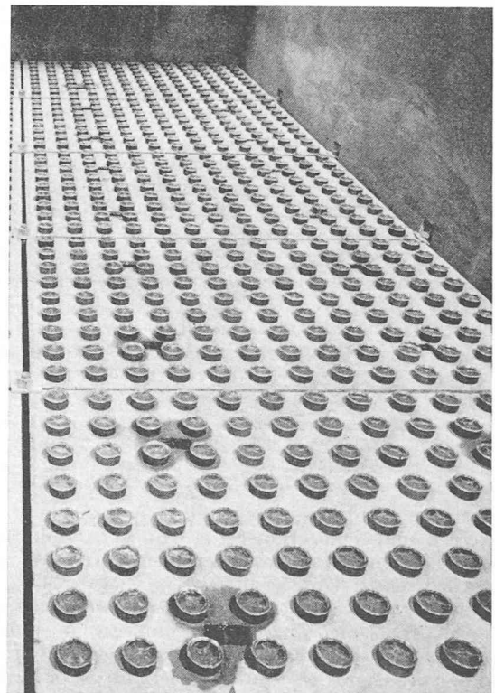
Fig. 3. — Fond filtrant terminé.
