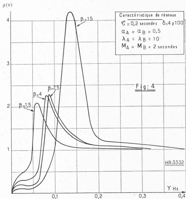
Fig. 4. — Exemple de caractéristiques harmoniques \frac{\Delta P_T}{\Delta \Pi_A} .
