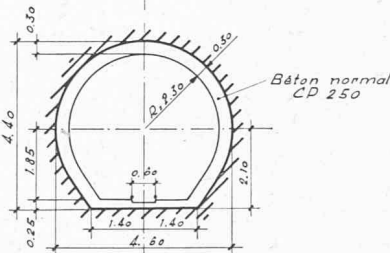
Fig. 3. Profils en travers type de la galerie et schémas d'injection
