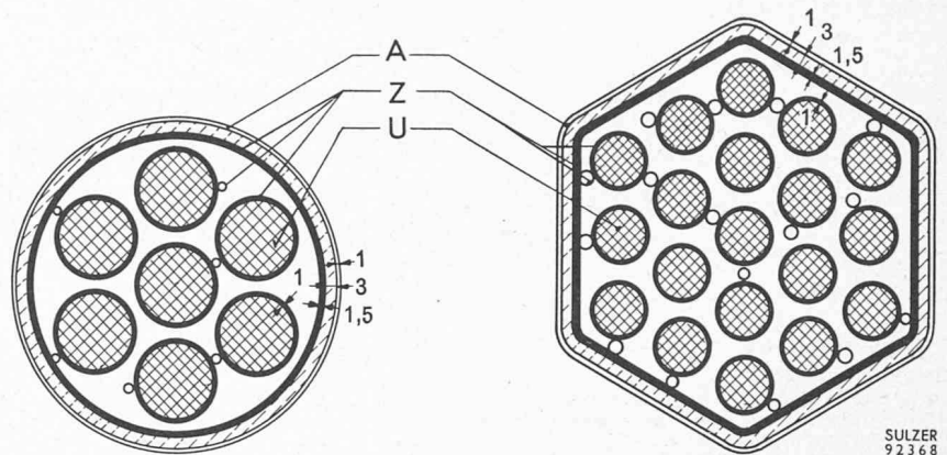
Fig. 1. — Données géométriques des éléments à groupes de barres.
