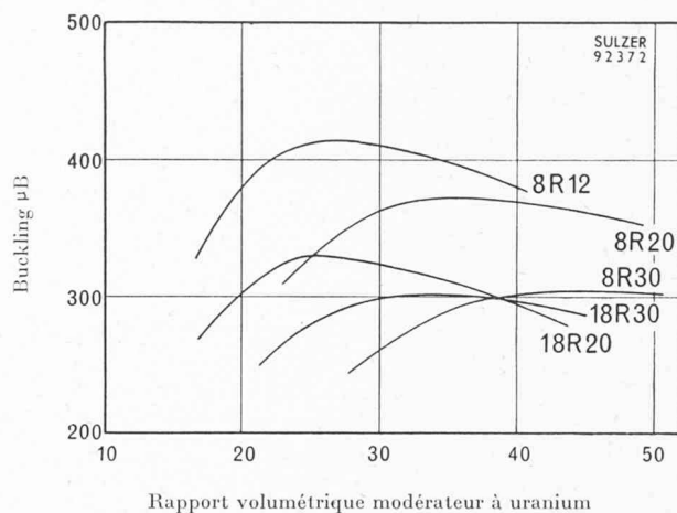
Fig. 6. — Buckling des éléments à groupes de tubes, à la puissance nominale.
