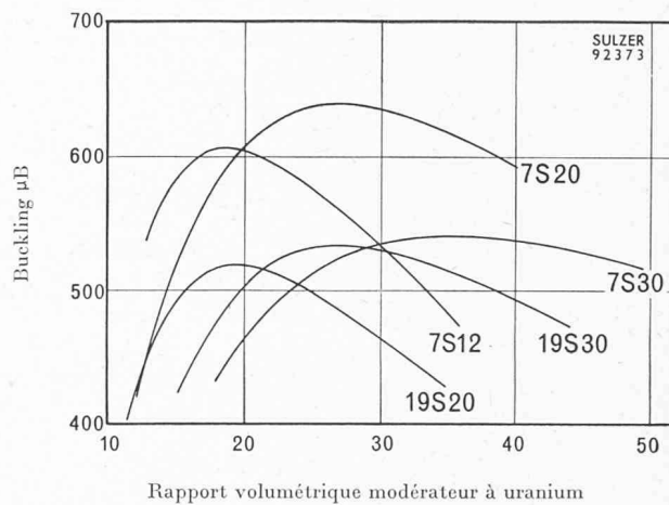
Fig. 7. — Buckling des éléments à groupes de barres, à la puissance zéro.
