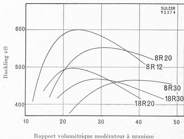
Fig. 8. — Buckling des éléments à groupes de tubes, à la puissance zéro.
