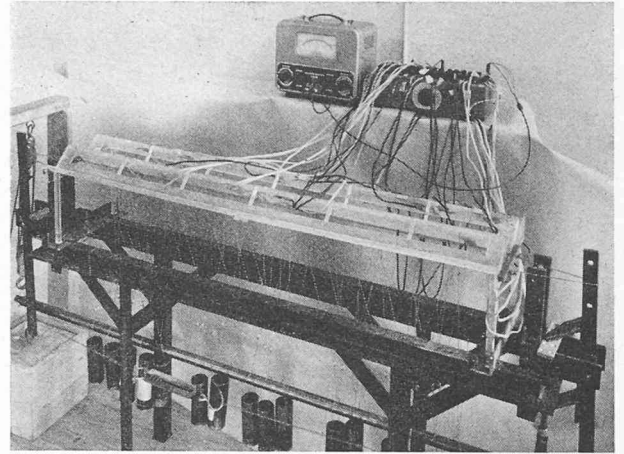
Fig. 6 a. — Modèle en plexiglas à l'échelle 1 : 25.
