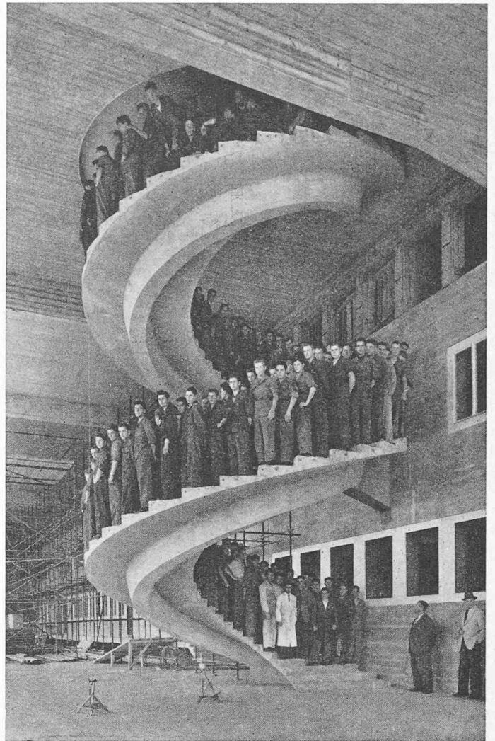
Fig. 2 a. — Escalier en spirale (B.B.C., Baden).
