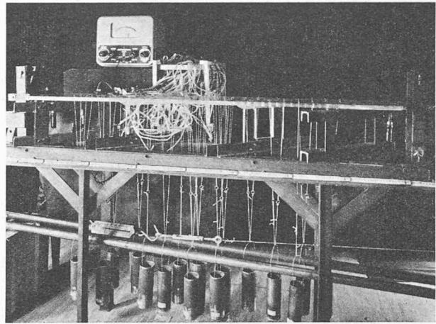
Fig. 5 b. — Modèle en plexiglas à l'échelle 1 : 40. Charges verticales et peson à ressort pour la mesure des efforts horizontaux.
