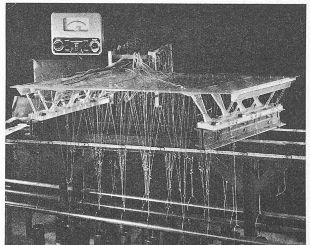
Fig. 7 a. — Modèle en plexiglas à l'échelle 1 : 50.
