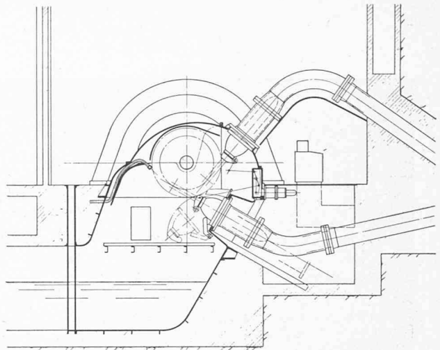
Fig. 9. — Adaptation d'injecteurs rectilignes sur turbine Pelton à double jet.
