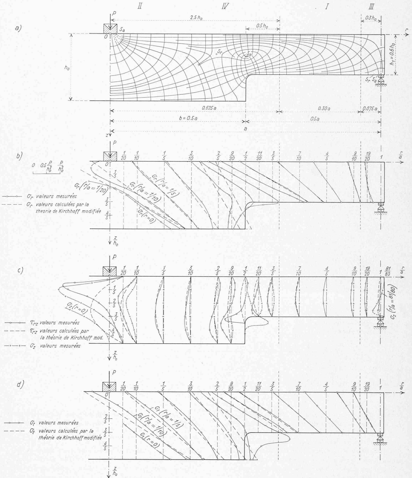
Fig. 7 a, b, c, d. — Modèle de la plaque figure 1 B. a) Trajectoires des tensions principales b), c), d) Diagrammes des tensions \sigma_r , \sigma_z , \tau_{rz} et \sigma_t .
