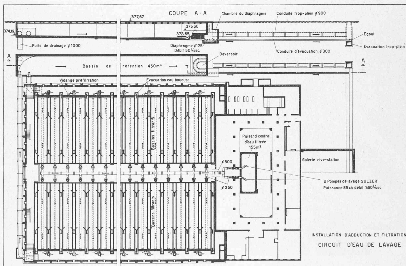
Fig. 21. — Coupes horizontale et verticale des bâtiments ; circuit d'évacuation des eaux de lavage.
